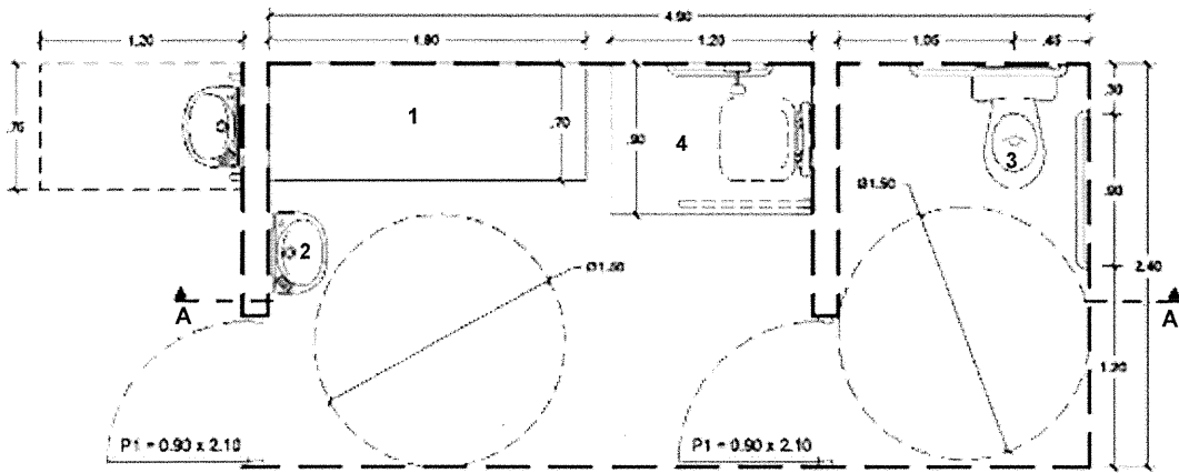
PLANTA
